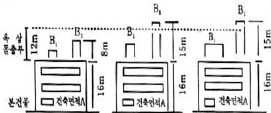
[그림 2-11] 옥상부분의 면적에 따른 건축물의 높이 산정
