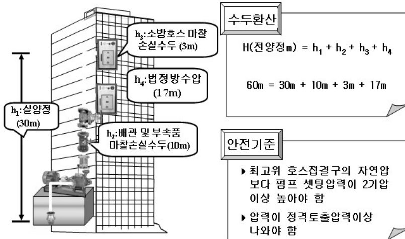
[그림 3-19] 양정계산과 압력설정
