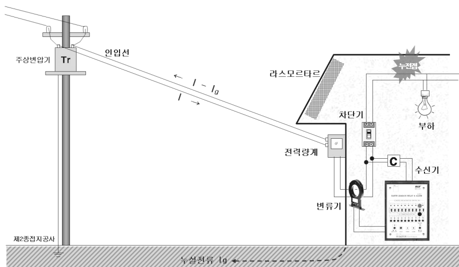
[그림 2-69] 누전경보기 설치구성도
