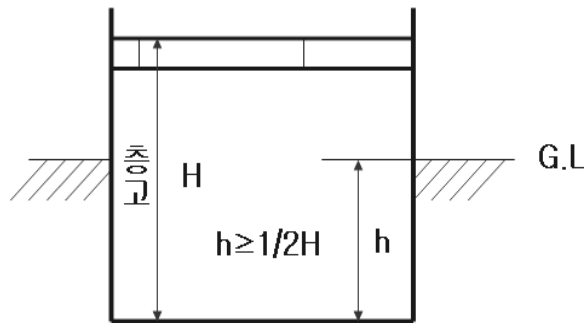
[그림 1-1] 지하층
