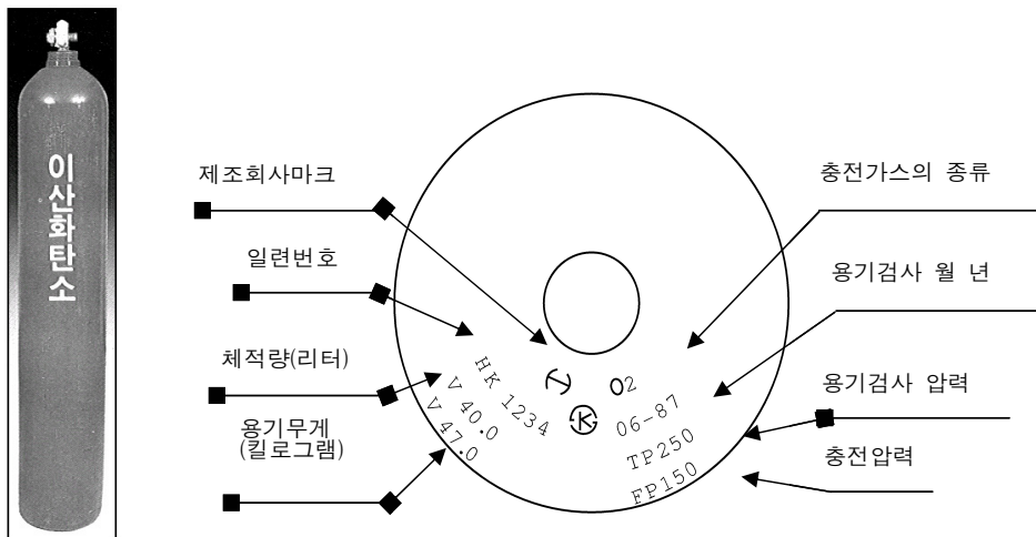
[그림 6-6] 가스저장용기
