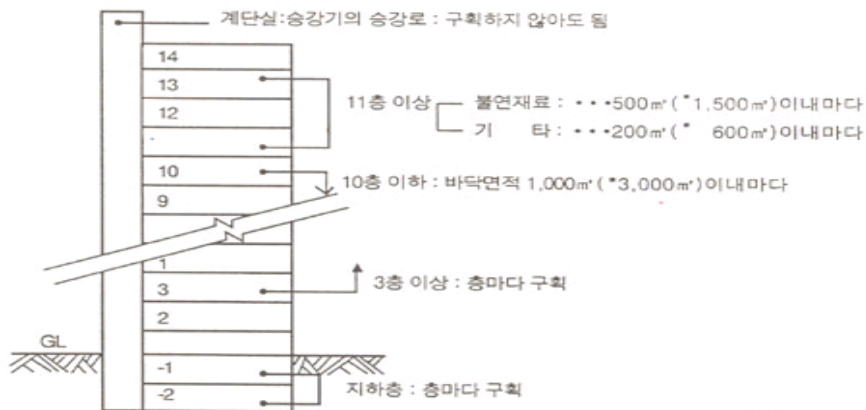
[그림 3-1] 방화구획 설치기준
