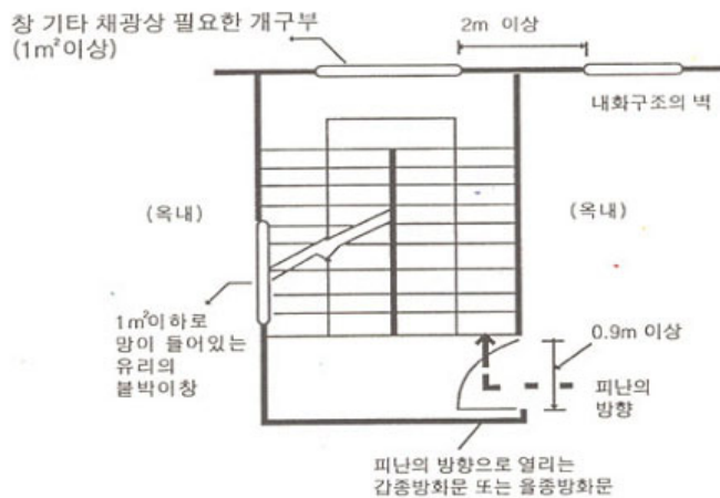
[그림 4-12] 옥내피난계단의 구조
