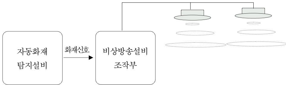
[그림 2-79] 비상방송설비의 작동흐름도
