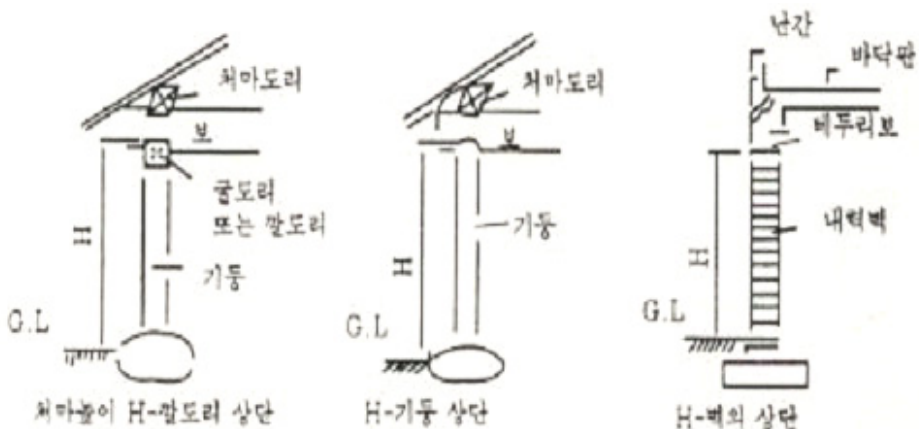
[그림 2-14] 처마높이 산정
