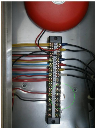
[그림 2-52] 중단저항 설치(발신기세트함 및 중단감지기)
