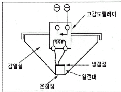
[그림 2-11] 열전대식감지기
