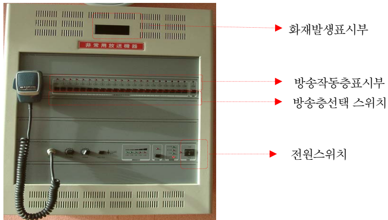
[그림 2-80] 비상방송설비의 스위치 및 표시등
