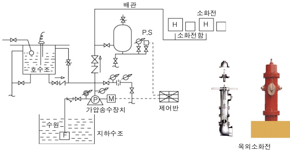
[그림 3-29] 옥외소화전 계통도
