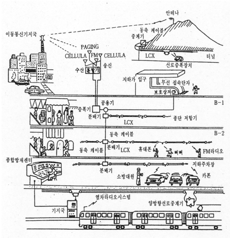
[그림 3-19] 무선통신보조설비의 사용
