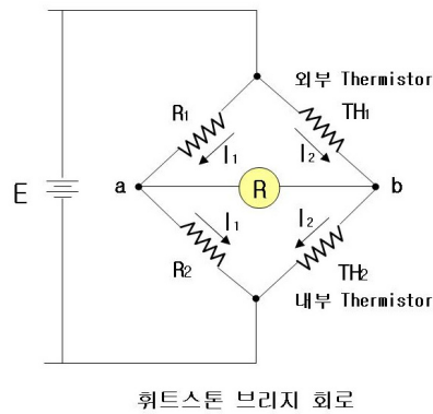
[그림 2-12] 열반도체식감지기
