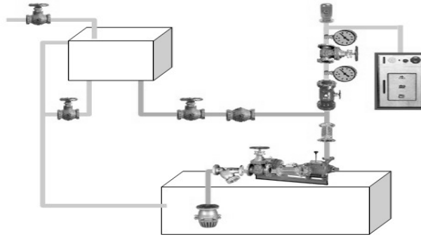
[그림 3-9] 물올림 장치 구조
