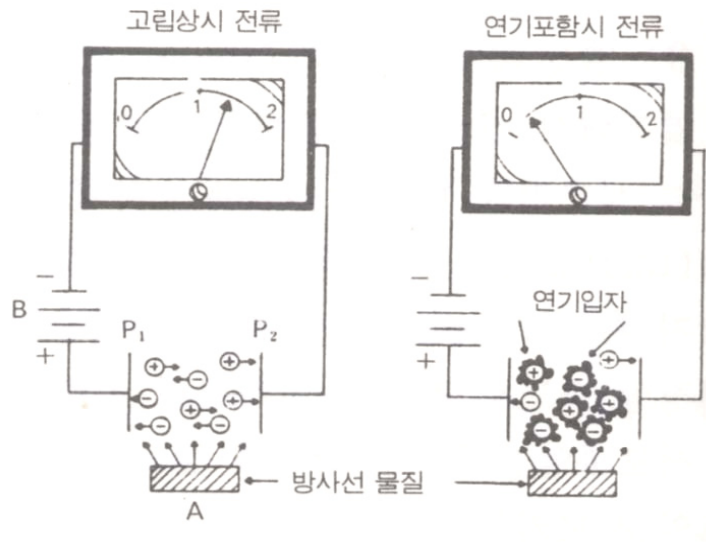
[그림 2-20] 이온화식감지기의 회로구성
