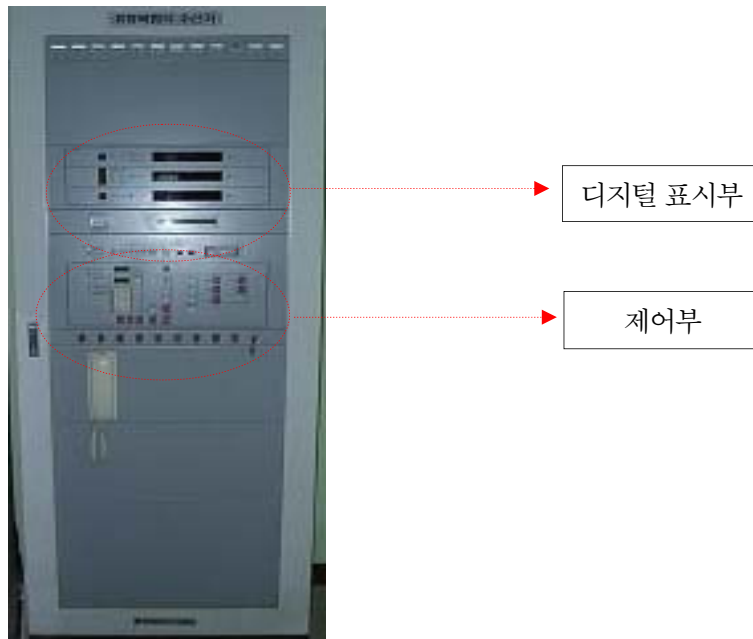
[그림 2-61] R형 수신기의 표시장치 및 제어부
