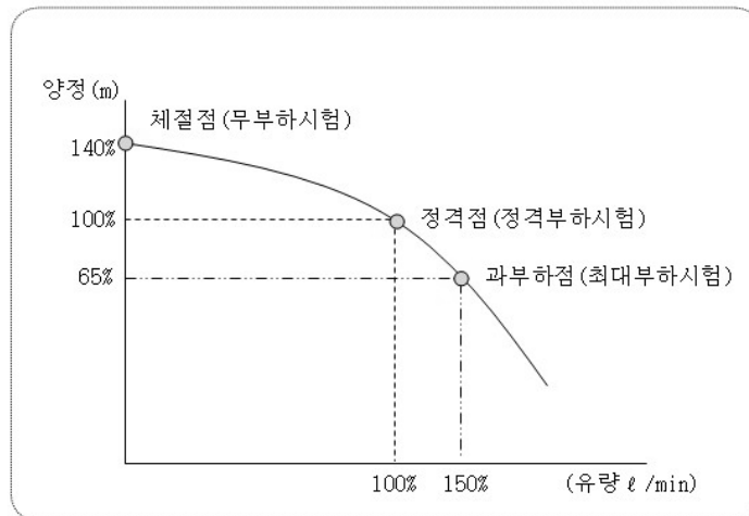
[소방펌프의 특성곡선]
