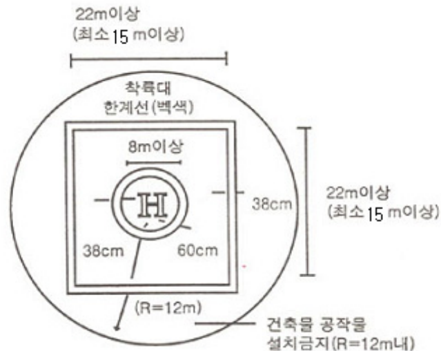
[그림 4-15] 헬리콥터의 설치기준
