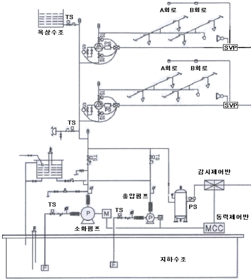
[그림 4-1] 준비작동식 스프링클러설비 계통도
