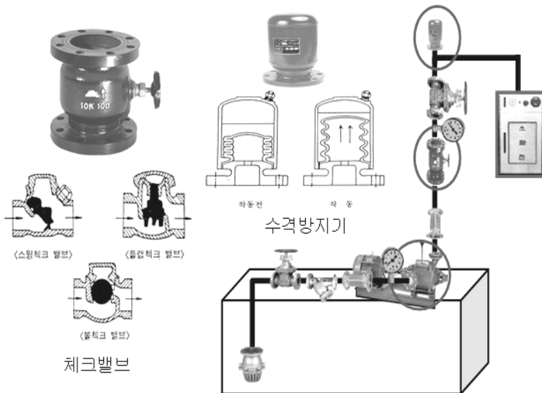
[그림 3-8] 체크밸브와 수격방지기
