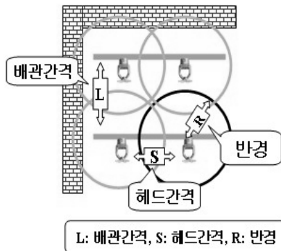
[그림 4-18] 정사각형 헤드배치 방법
