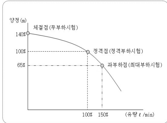
[소방펌프의 특성곡선]
