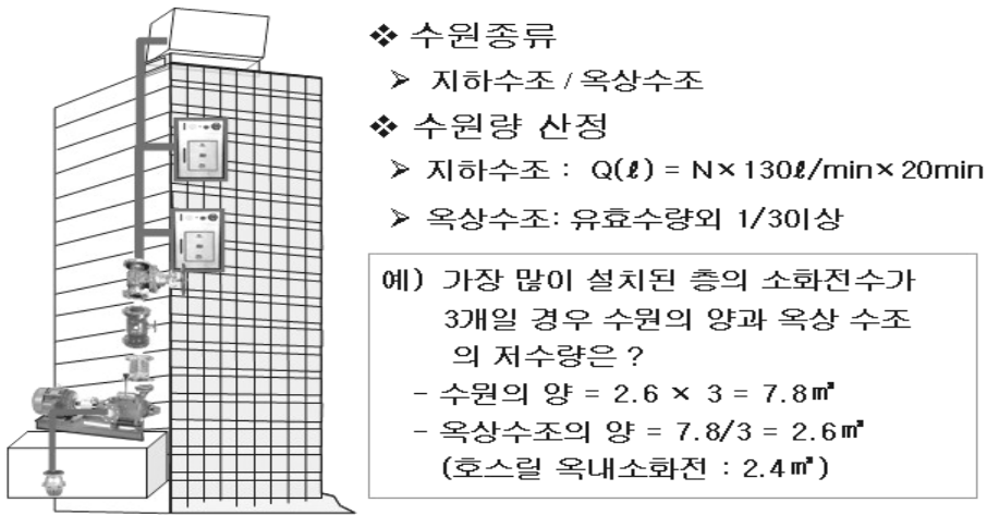
[그림 3-2] 옥내소화전 수원산정
