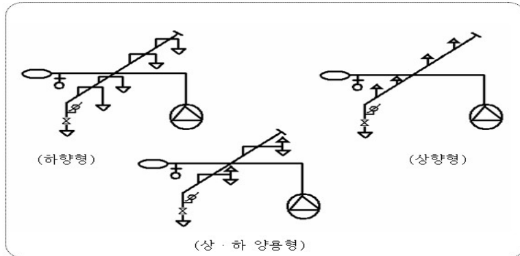
[그림 4-17] 헤드설치방법
