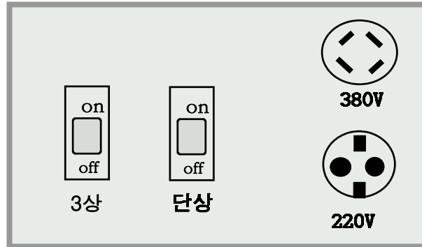
[그림 3-18] 비상콘센트함
