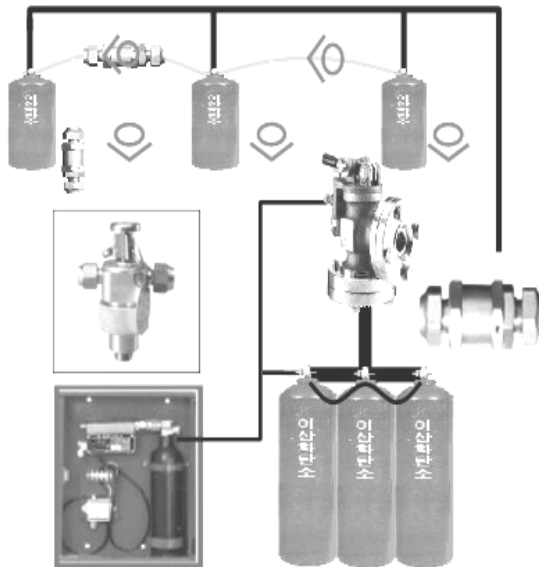
[그림 6-11] 저장용기 점검
