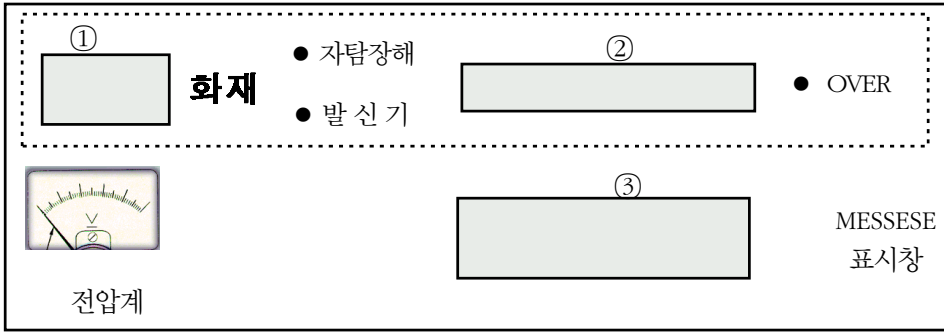
[그림 2-62] 표시부
