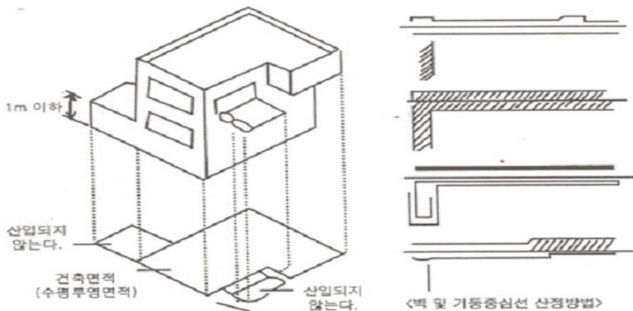
[그림 2-4] 건축면적의 산정방법
