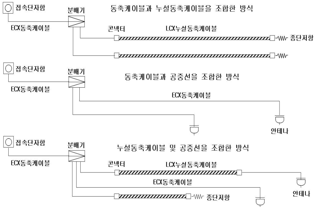
[그림 3-23] 무선통신보조설비의 종류
