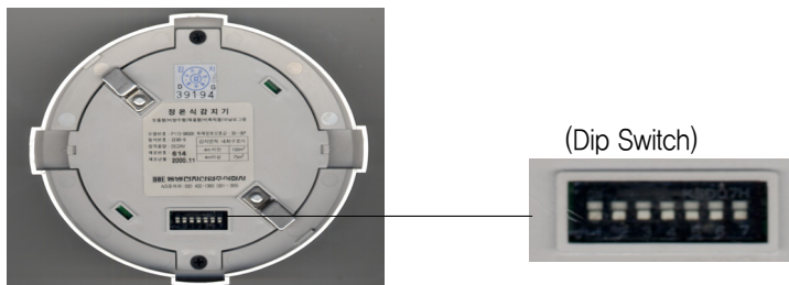
[그림 2-30] 주소형감지기의 주소지정
