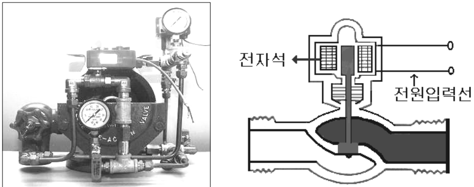
[그림 4-7] 밸브와 솔레노이드
