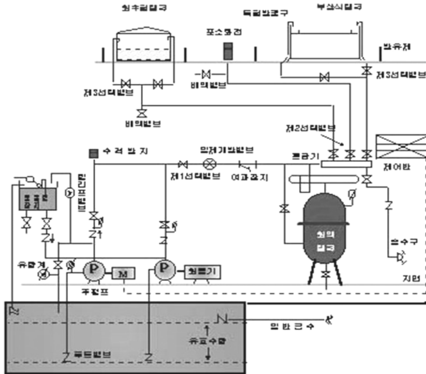
[그림 5-12] 고정포방출설비
