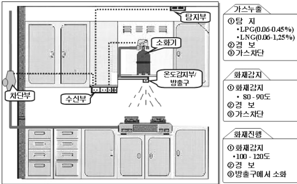
[그림 2-6] 주방용자동소화장치
