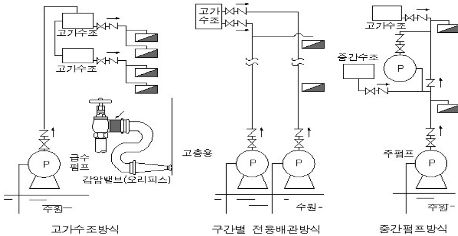
[그림 3-21] 감압방식
