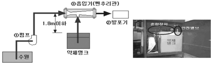
[그림 5-6] 라인프로포셔너 방식
