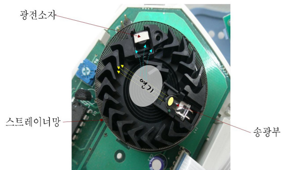
[그림 2-23] 산란광식의 내부
