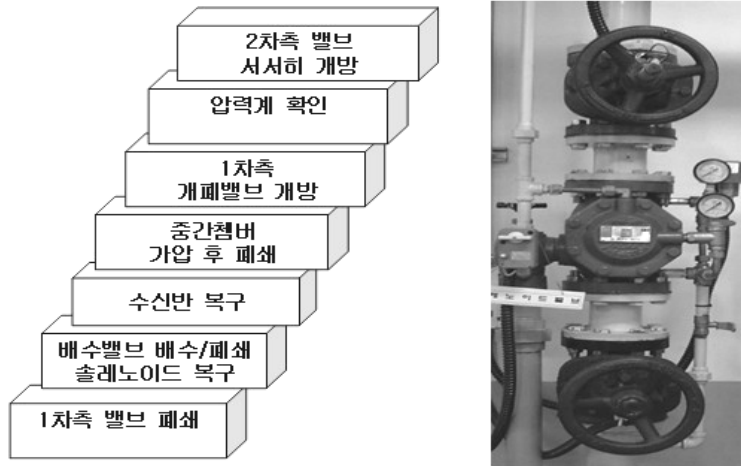
[그림 4-29] 준비작동식 복구순서
