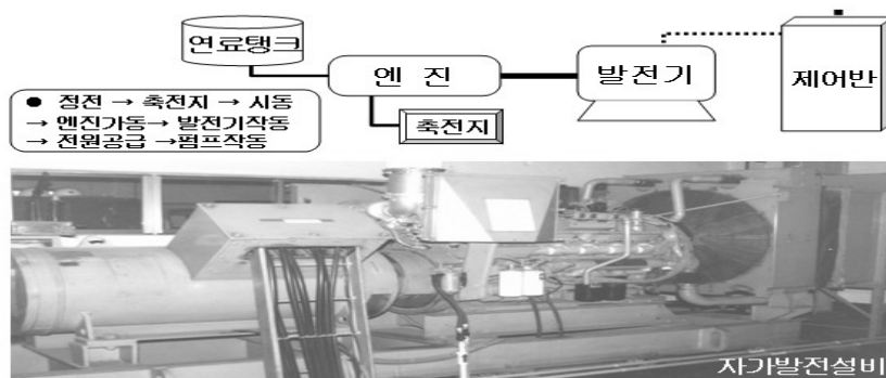
[그림 3-27] 자가발전설비
