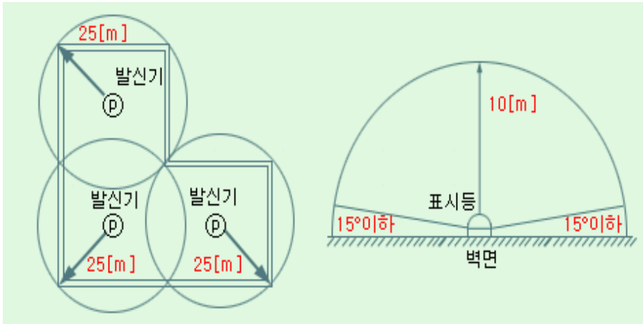
[그림 2-39] 발신기의 설치거리
