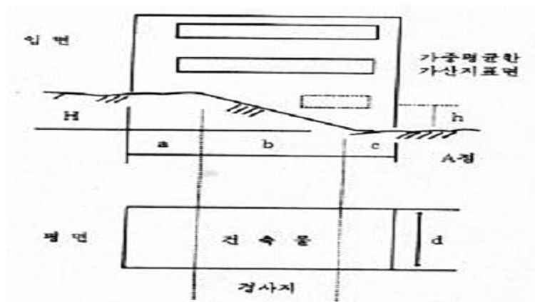
[그림 2-9] 지표면의 산정
