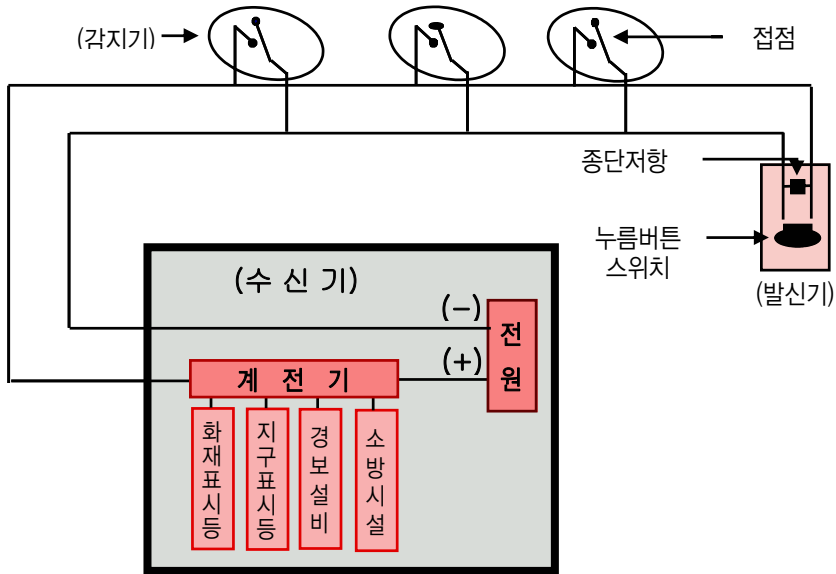
[그림 2-2] 자동화재탐지설비의 회로 간략도
