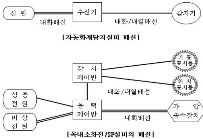
[그림 3-26] 소방시설별 내화/내열배선 방식
