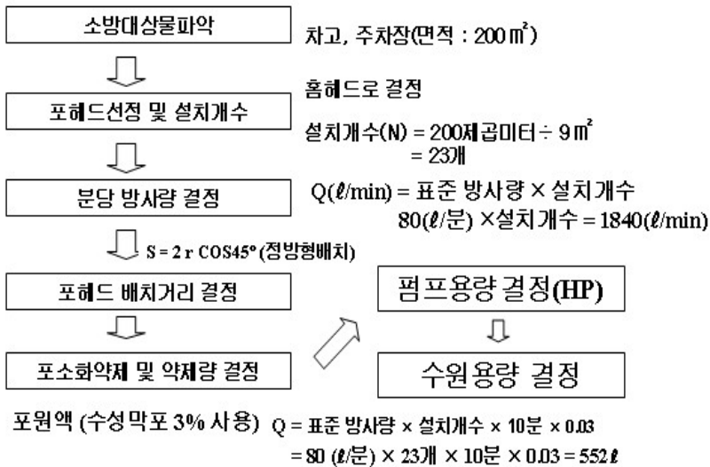
[그림 5-23] 홈헤드 설계방식 검토
