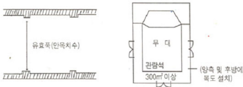
[그림 4-8] 복도의 유효너비 및 설치기준
