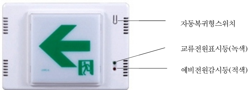
[그림 3-12] 유도등의 표시등 및 스위치
