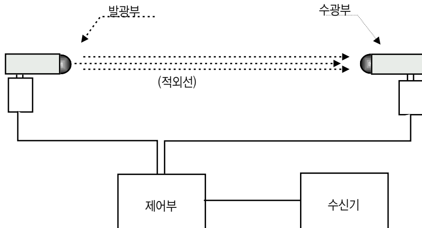
[그림 2-24] 광전식분리형감지기
