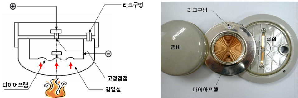
[그림 2-4] 차동식스포츠형 감지기 구조
