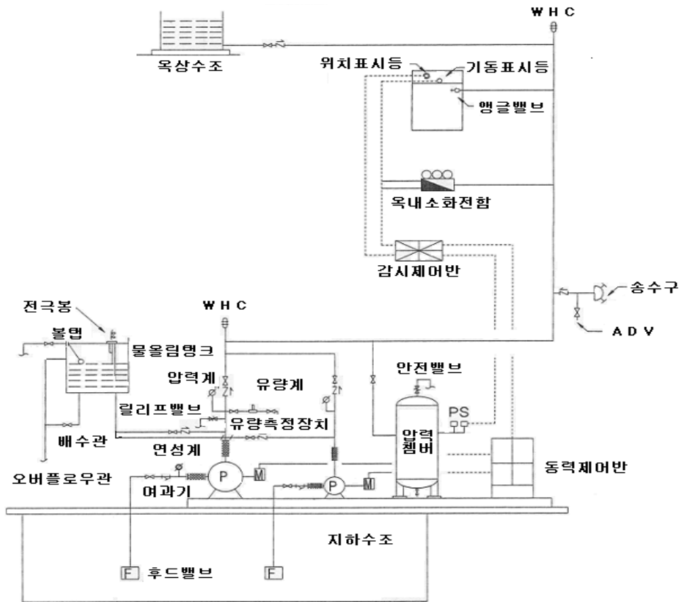
[그림 3-1] 옥내소화전 계통도 6)
