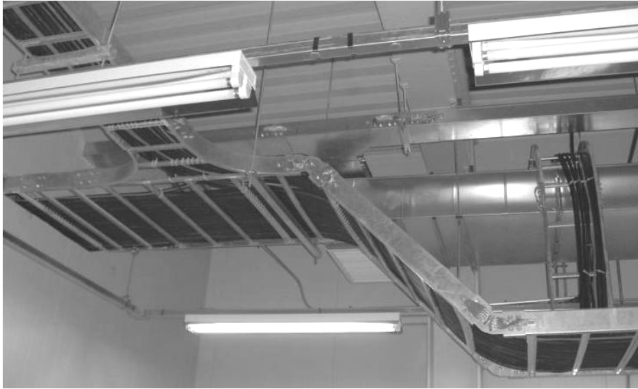
[그림 5-5] 케이블공사
