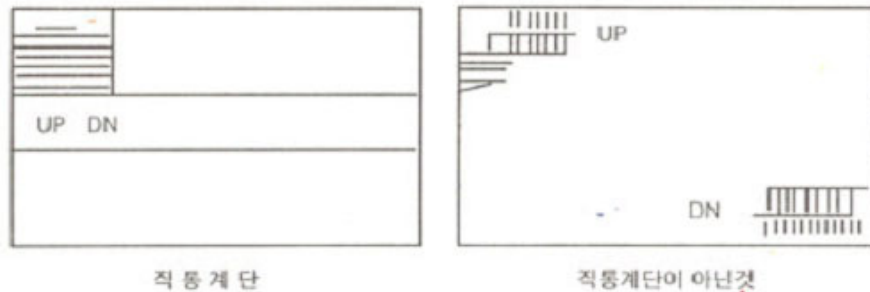
[그림 4-3] 직통계단
