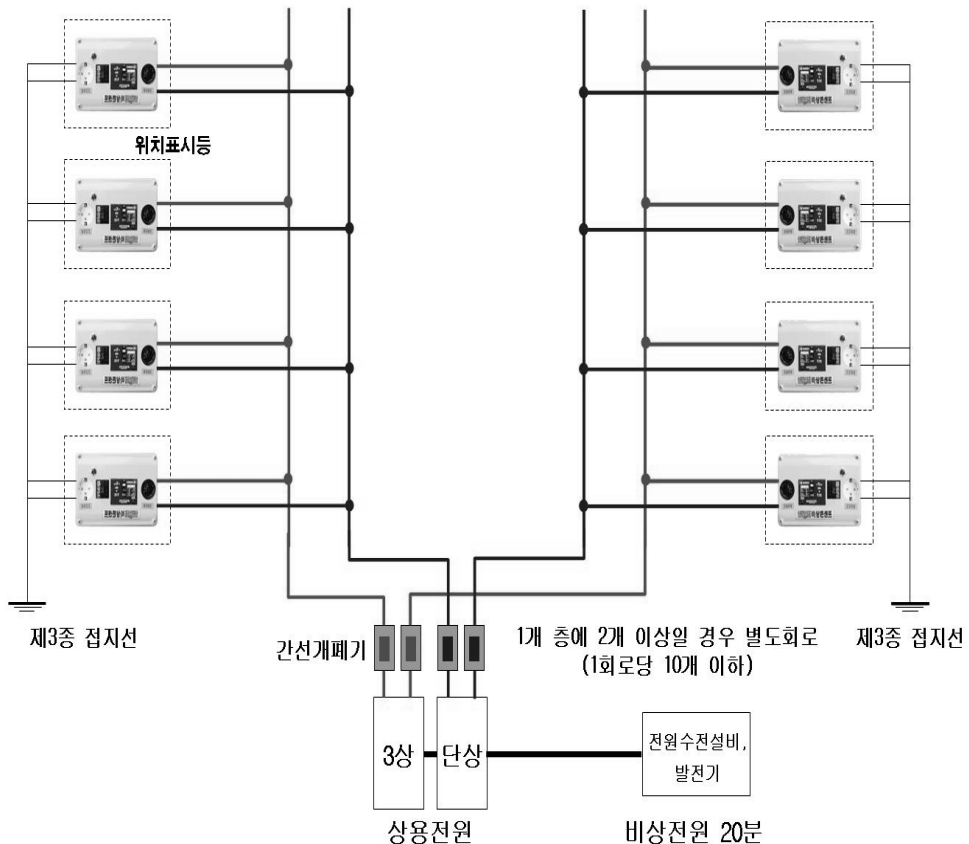
[그림 3-16] 비상콘센트설비의 배선도
