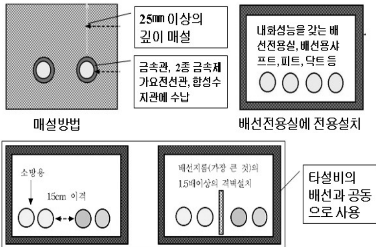
[그림 3-25] 내화배선 공사방법
