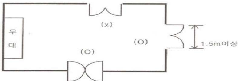
[그림 4-5] 출구의 문 설치기준
