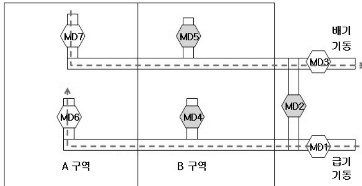
[그림 7-4] 화재시 제연설비로 전환
