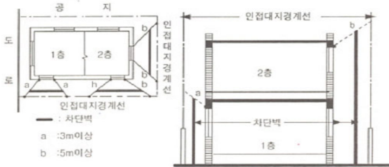
[그림 3-4] 차단벽 설치
