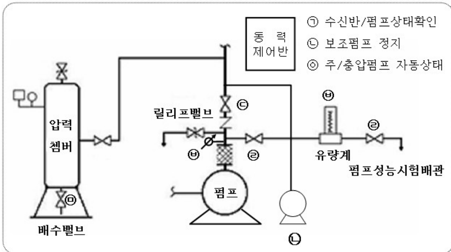
[그림 3-16] 펌프성능시험 방법
