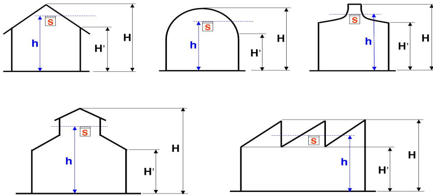
[그림 2-31] 건축물별 감지기의 설치높이 산정방법
