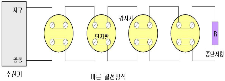
[그림 2-53] 감지기 배선 송배선방식
