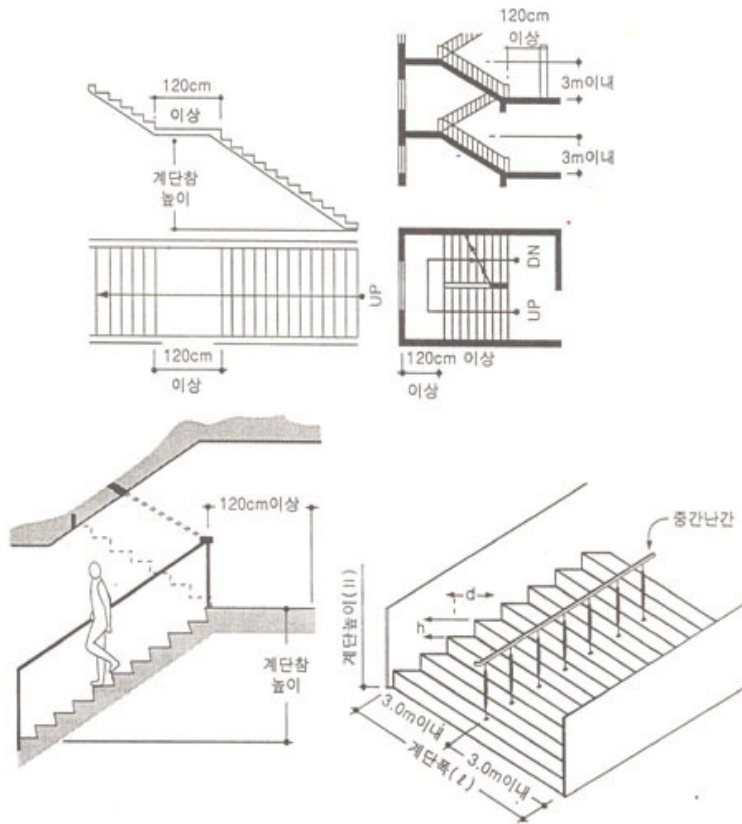
[그림 4-9] 계단의 설치기준
