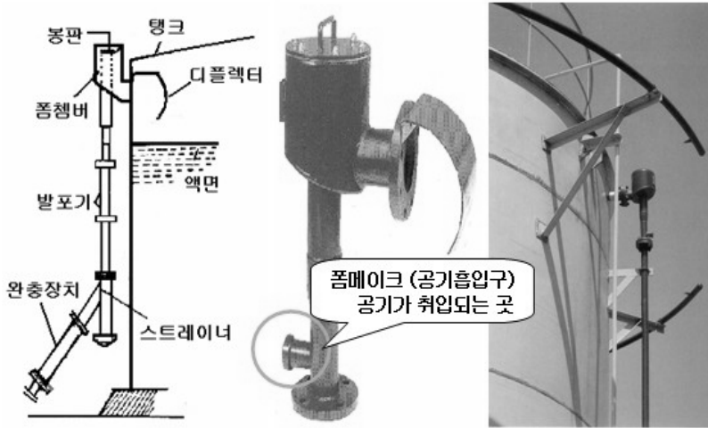
[그림 5-15] II형 방출구
