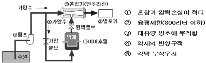
[그림 5-8] 격막이 있는 방식
