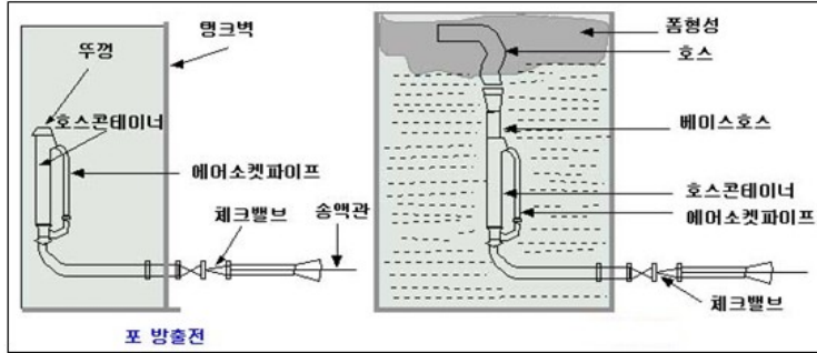
[그림 5-18] 반표면하 방식
