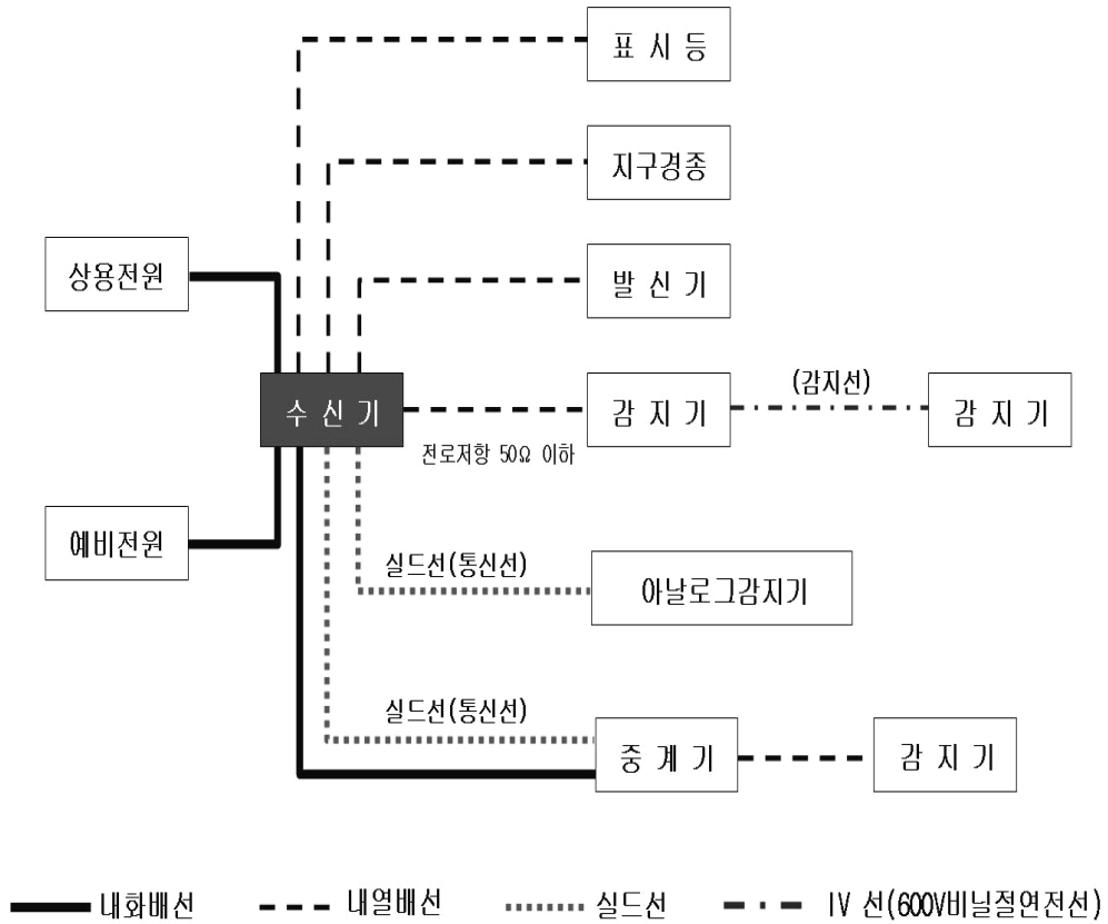
[그림 5-7] 자동화재탐지설비 구간배선
