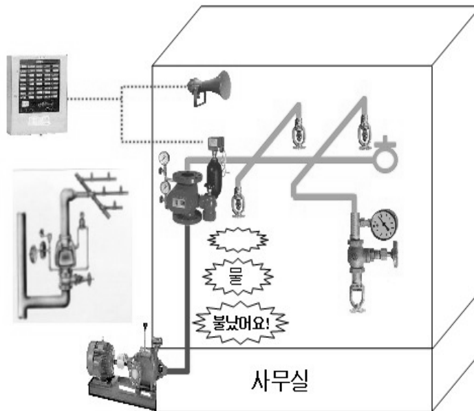
[그림 4-2] 스프링클러설비 구조 및 작동
