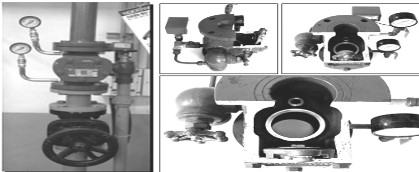
[그림 4-3] 습식벨브 구조
