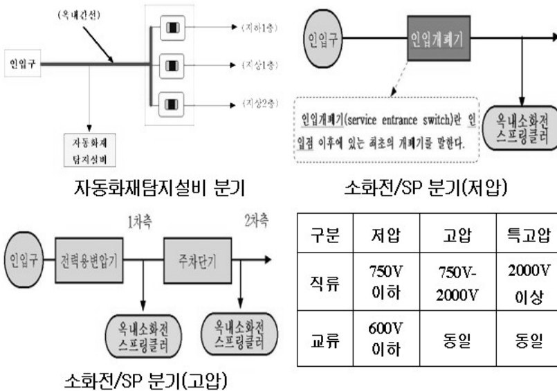
[그림 3-24] 상용전원 분기방식
