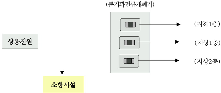
[그림 5-3] 소방시설 상용전원의 분기(○)
