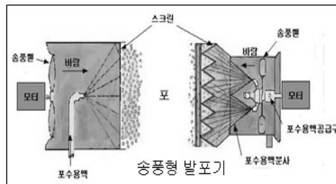
[그림 5-20] 흡출형/송풍형 고발포기
