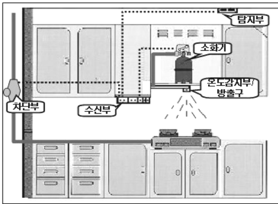
[그림 2-12] 주방용자동소화장치 점검
