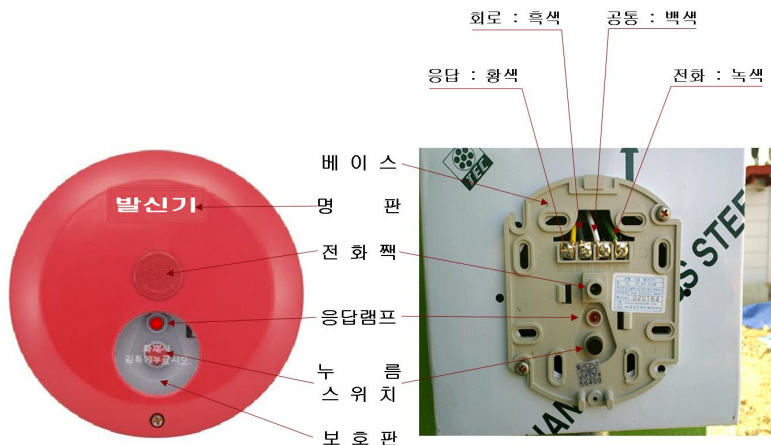
[그림 2-38] 발신기 구성
